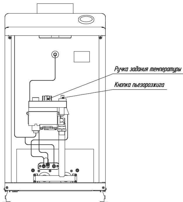
Рисунок 6 - Особенности котла с газовым блоком 710 MINISIT.
