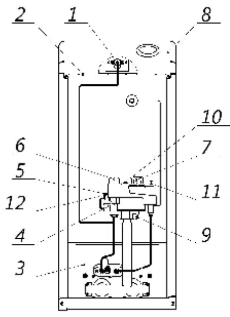
Рисунок 2 - Устройство котла с газовым блоком автоматики САБК-АТ
