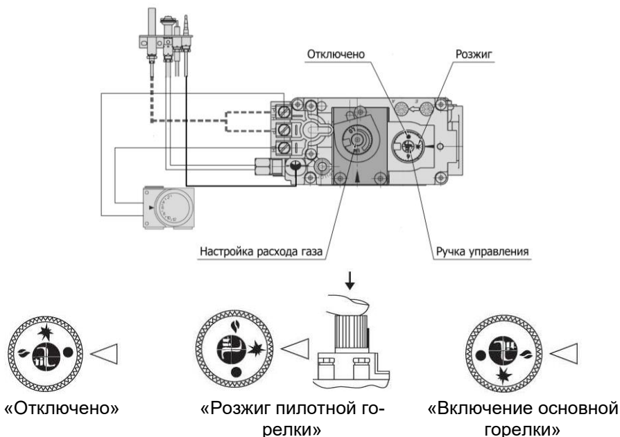
Рисунок 3 - Элементы управления на газовом блоке 820 NOVA mV.
