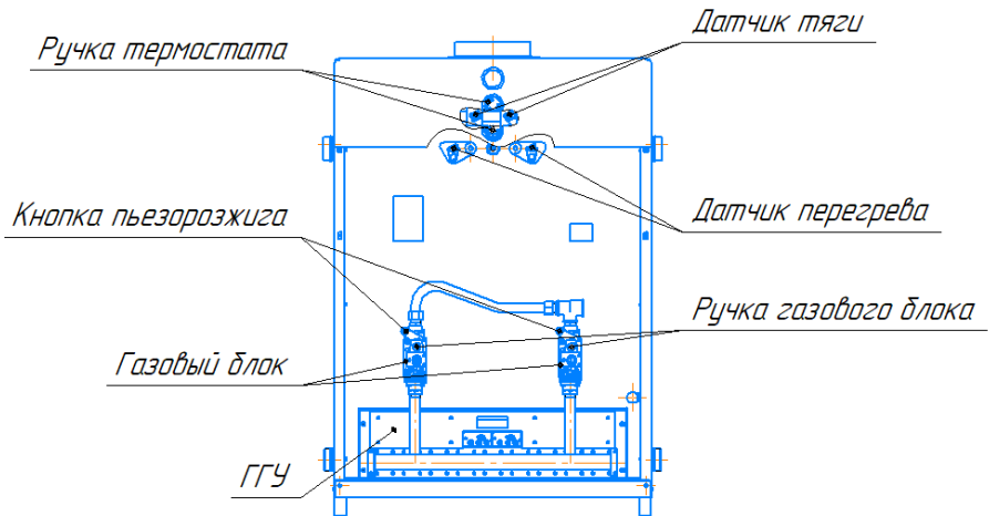
Рисунок 4 - Особенности аппарата с двумя газовыми блоками 820 NOVA mV.
